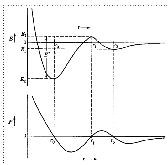
Slika 2. Promena potencijalne energije i sile pri uzajamnom dejstvu dva atoma /15/
